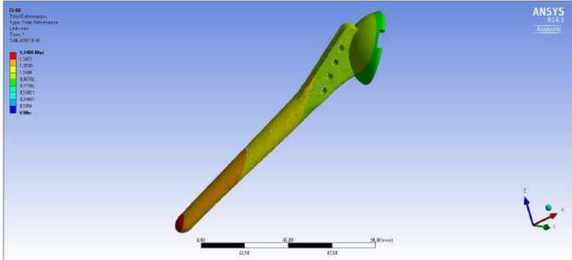
Şekil 3.153. Kol 60° abdüksiyondayken humeral saptaki yerdeğişim analizi lateral görünüm
