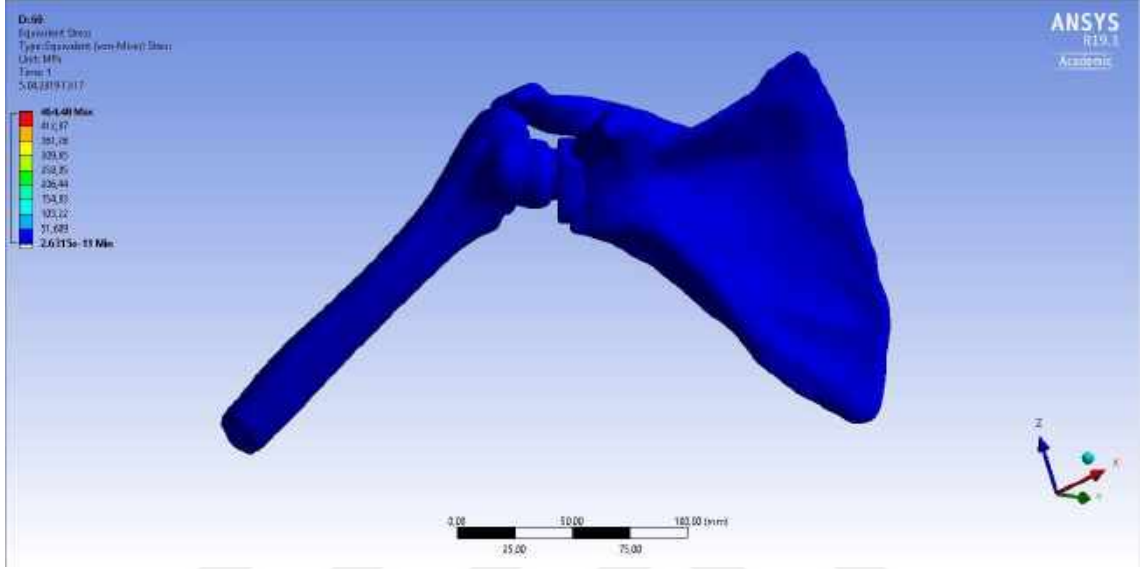
Şekil 3.76. 60° abdüksiyondayken Omuz modelinde Von Misses Eşdeğer stres dağılımı Humeral Sap
