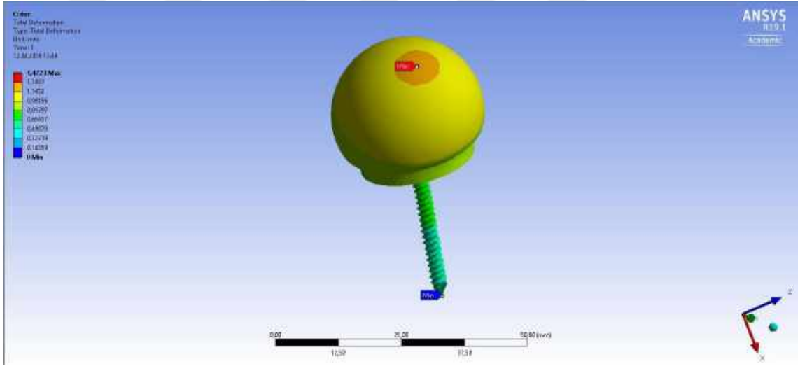
Şekil 3.115. Humeral kürede yer değiştirme II
