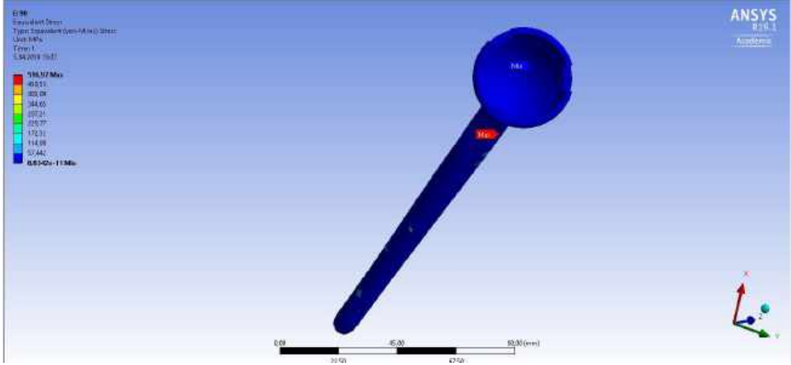
Şekil 3.91. Kol 90° abdükiyodayken humeral sapta Von Misses Eşdeğer Stres Analizi (medial)
