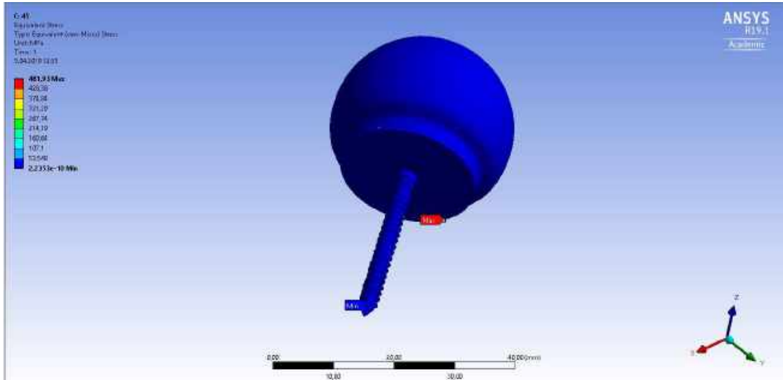
Şekil 3.68. Kol 45° abduksiyundayken Glenosferde Von Misses Eşdeğer Stres (Inferior)
