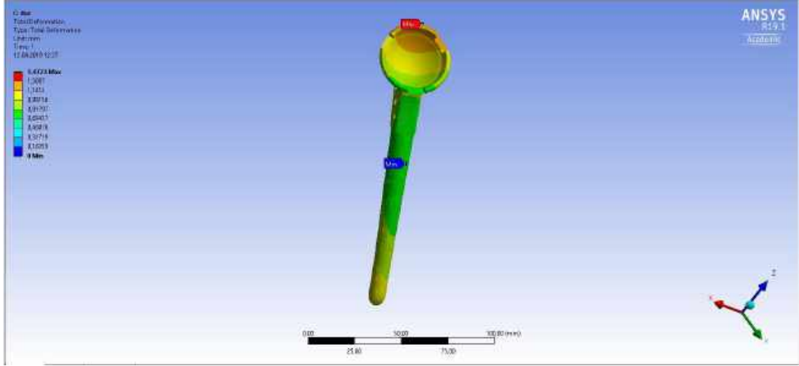
Şekil 3.110. Humeral Sapta toplam yerdeğiştirme III
