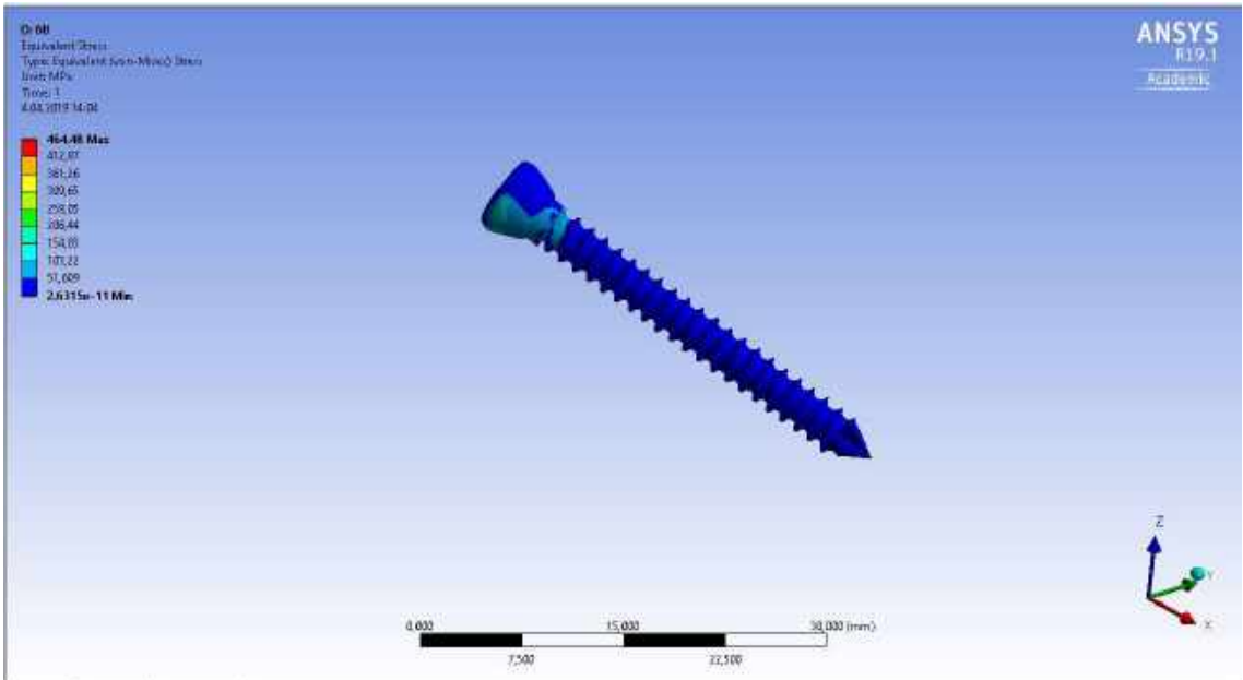
Şekil 3.85. 60° abdüksiyondayken I. çivideki Gerilme analizi
