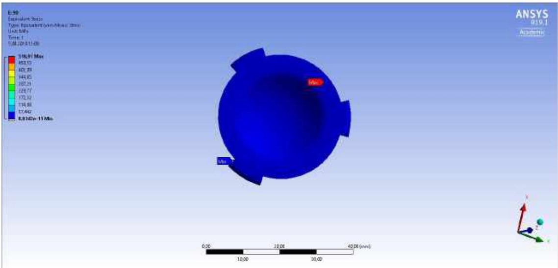
Şekil 3.92. Kol 90° abdükiyodayken humeral kapta Von Misses Eşdeğer Stres Analizi (Anterior)
