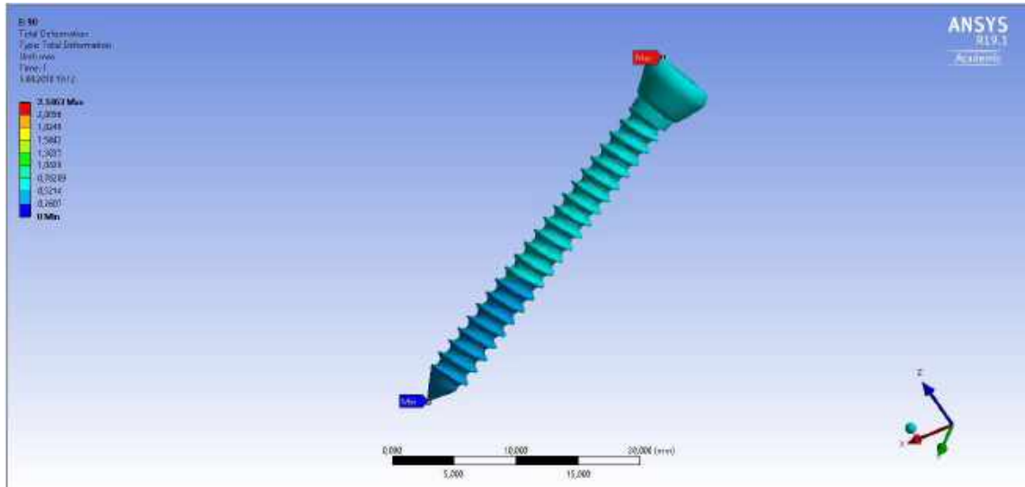
Şekil 3.174. 90° abdukte kolda II. Çivide yerdeğiştirme analizi
