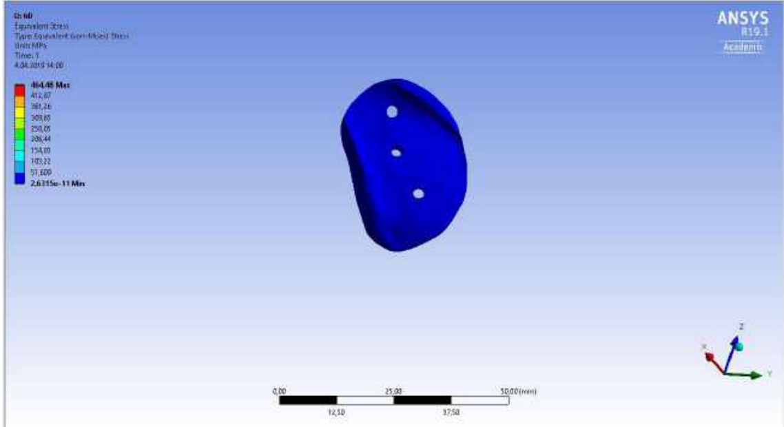
Şekil 3.84. 60° abdüksiyondayken taban palakasında Gerilme analizi (Anterior)
