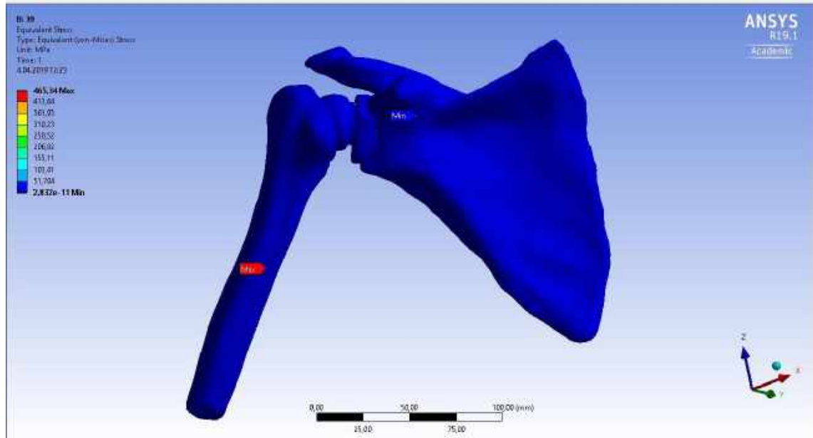
Şekil 3.51. Kolun 30° abdüksiyon hareketinde Von Misses Eşdeğer Stres Dağılımı
