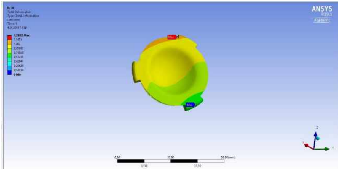
Şekil 3.130. Kol 30° abdüksiyondayken UHMWPE humeral kapda yerdeğitirme
