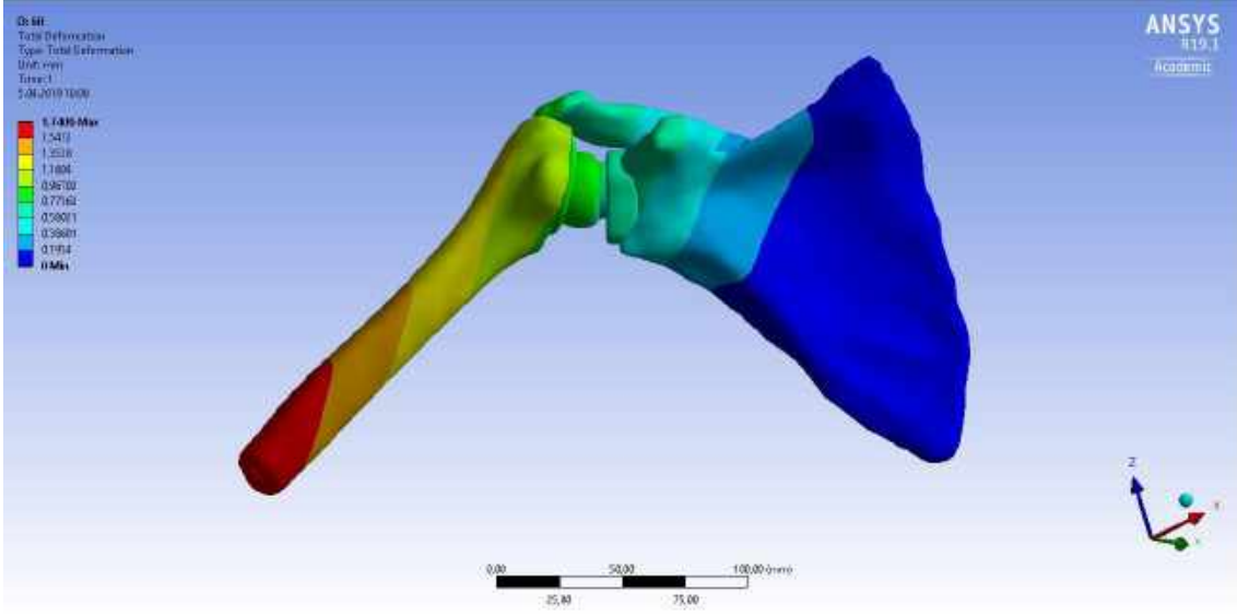
Şekil 3.152. Kolun 60° abdüksiyonunda yerdeğiştirme analizi sonuçları
