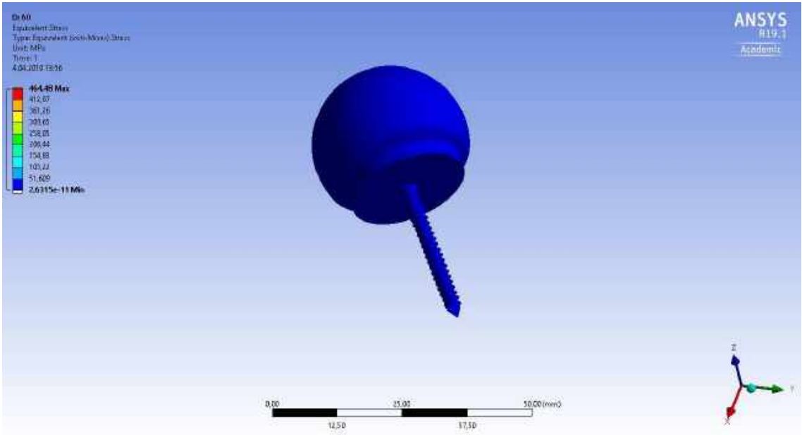
Şekil 3.81. 60° abdüksiyondayken glenosferde Gerilme analizi (Inferior)
