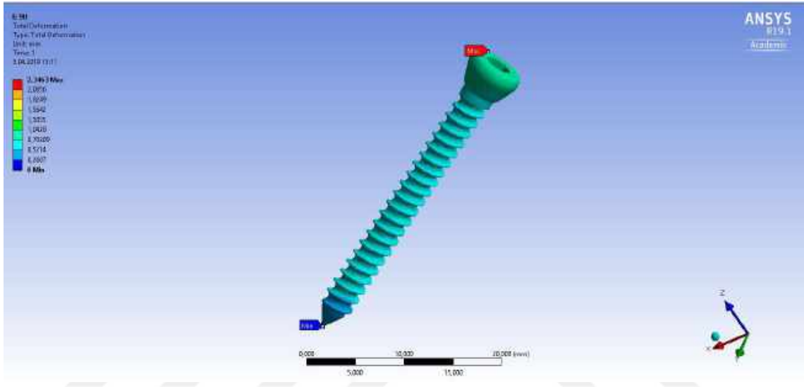
Şekil 3.173. 90° abdukte kolda I. Çivide yerdeğiştirme analizi
