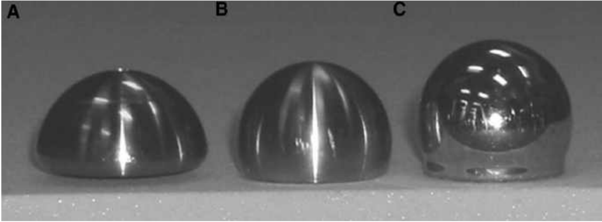
Şekil 2.50. Delta III (A), RSP-r (B) RSP-nötral (C) glenoküreler; lateral offset (taban plaktan glenoküre ile polietilen kap arasındaki eklemel temasa olan uzaklık) sırasıyla 16, 23 ve 27 mm. [45]
