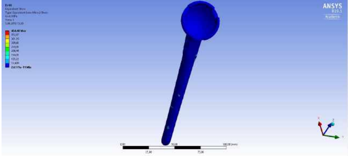
Şekil 3.78. 60° abduksiyondayken Humeral Sapın Gerilme analizi (Medial)
