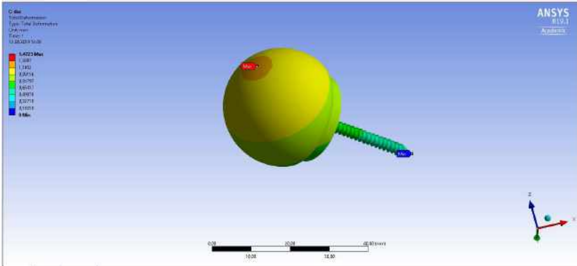
Şekil 3.113. Humeral kürede yer değiştirme I
