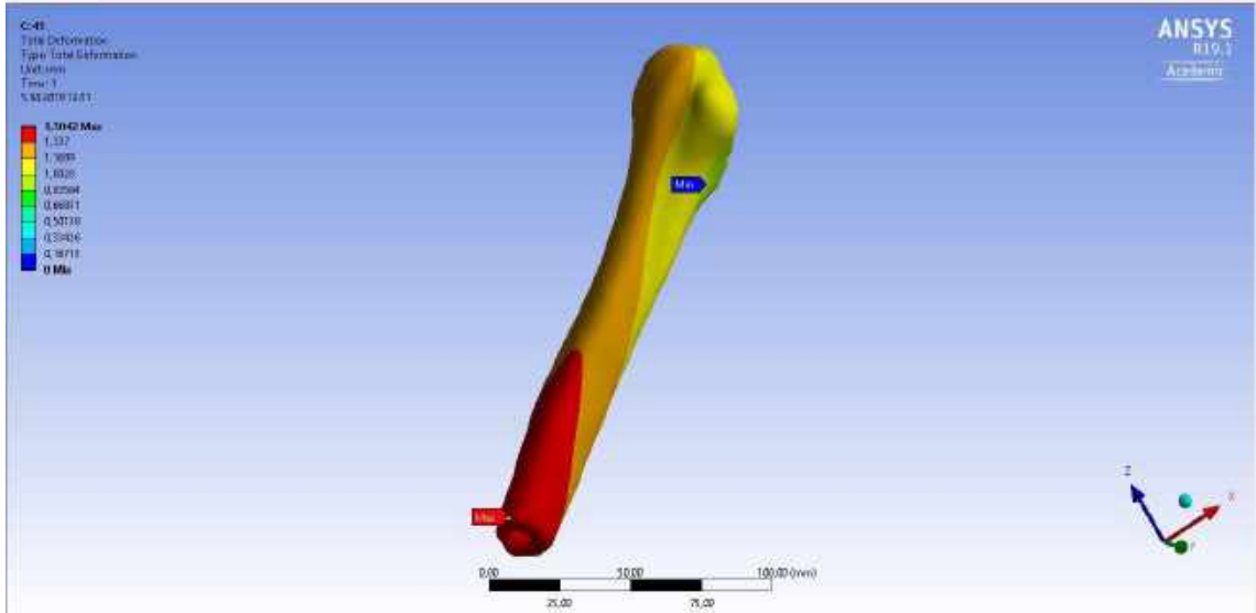
Şekil 3.150. 45° abdukte kolda humerusun yerdeđiştirme analizi posterior görünüm
