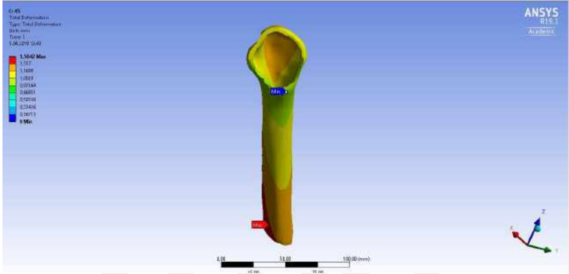
Şekil 3.149. 45° abdukte kolda humerusun yerdeđiştirme analizi anterior görünüm
