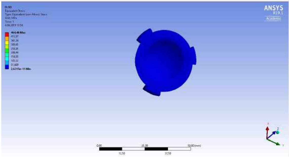
Şekil 3.79. 60° abduksiyondayken UHMWPE Humeral Kapta Gerilme analizi (Anterior)
