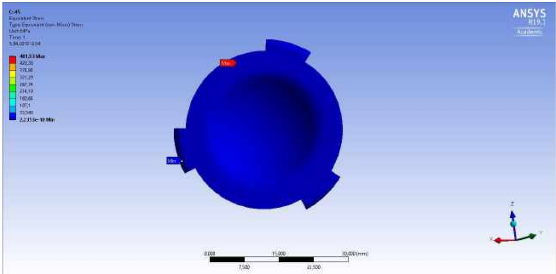
Şekil 3.66. Kol 45° abdüksiyondayken Humeral Kapta Eşdeğer Stres (Anterior)
