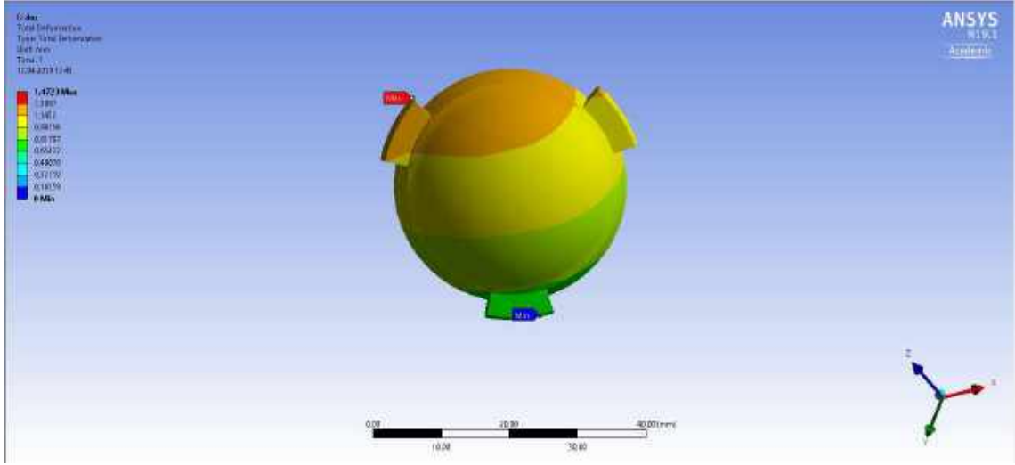
Şekil 3.112. UHMWPE Humeral Kaptı Yerdeğiştirme Analizi Posterior
